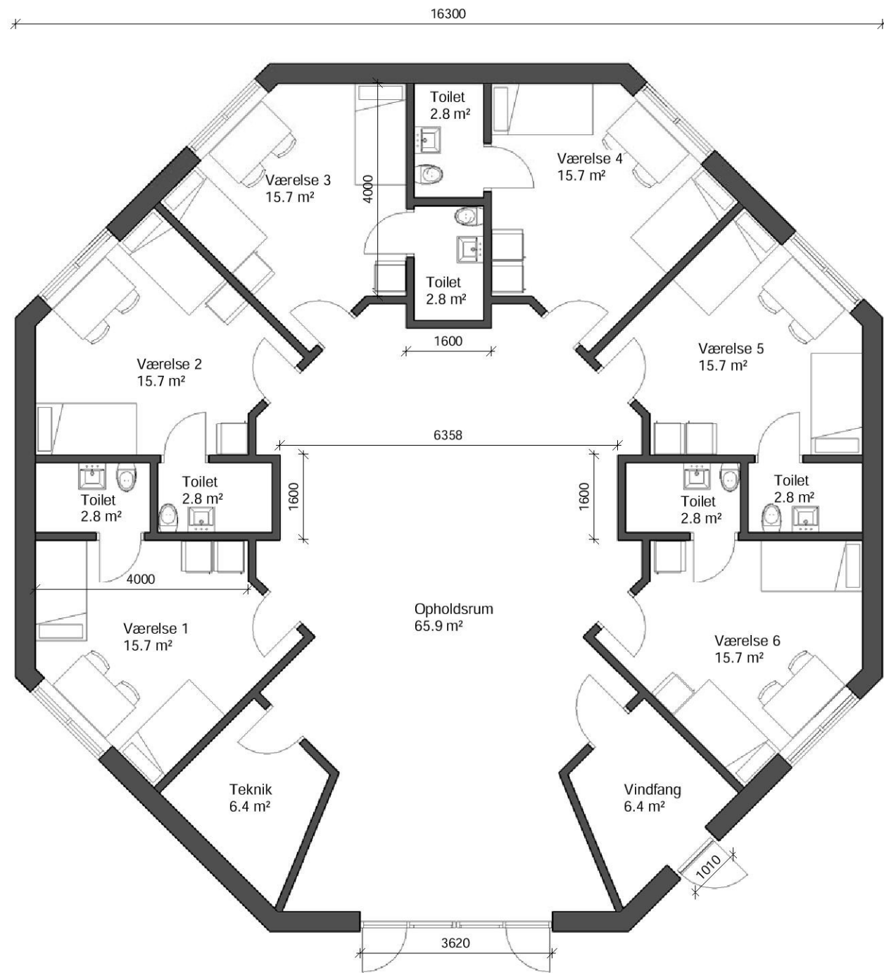
(01) Stueplan M16 1 : 100
