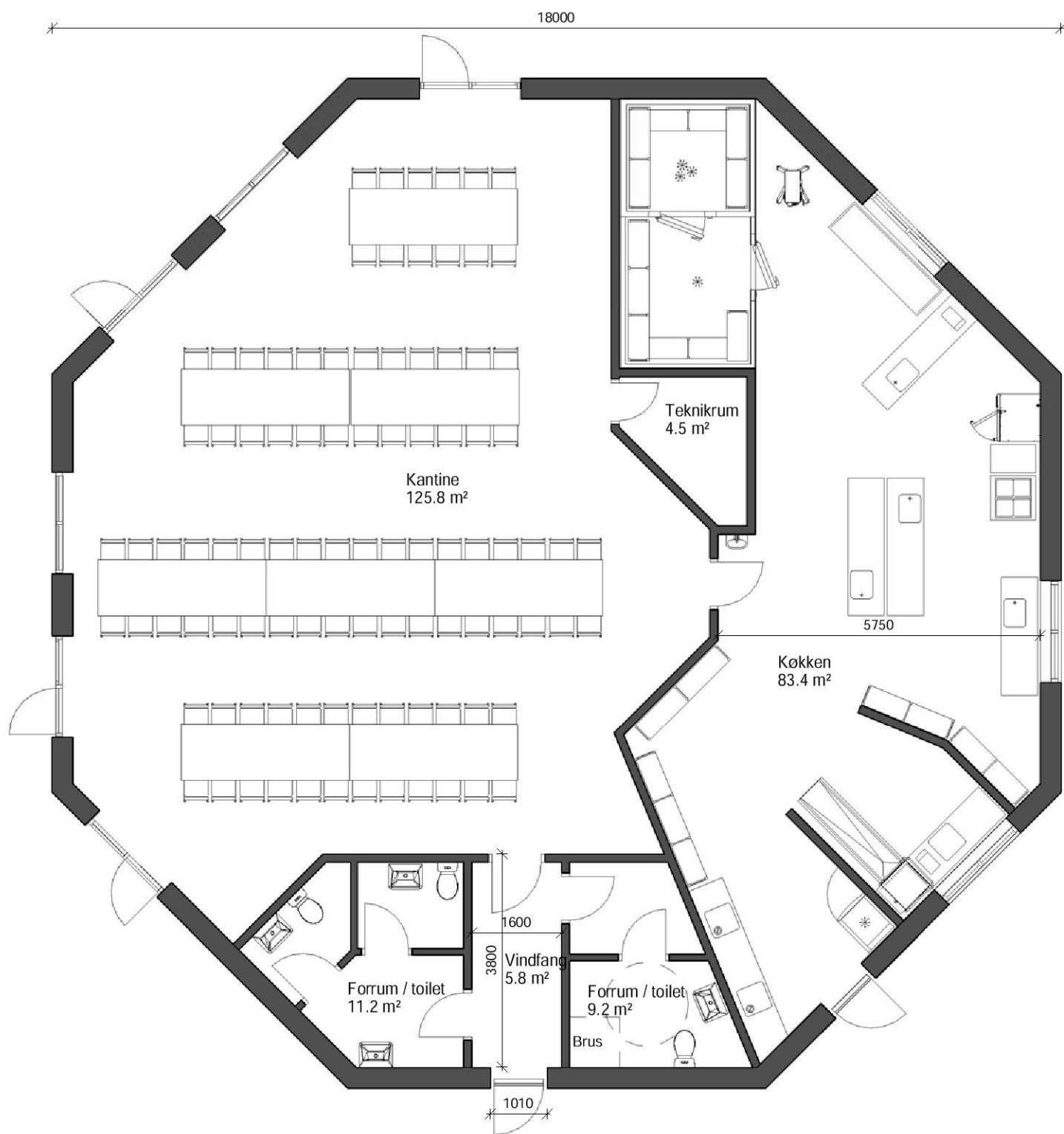
(01) Stueplan Kantine_M18 1 : 100
